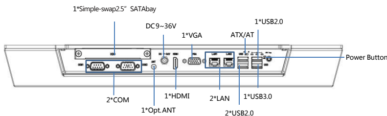
该图是去掉IO盖板后的2D图
